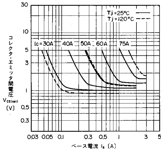
出力特性
