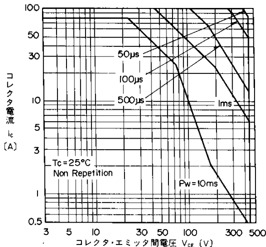
安全動作領域特性(非繰返し)
